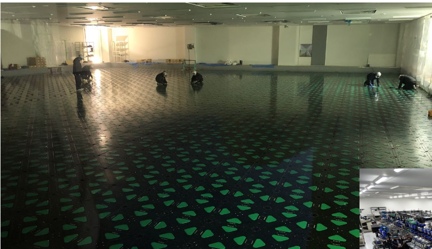
山形カシオ新工場 時計製造フロアの防震システム
